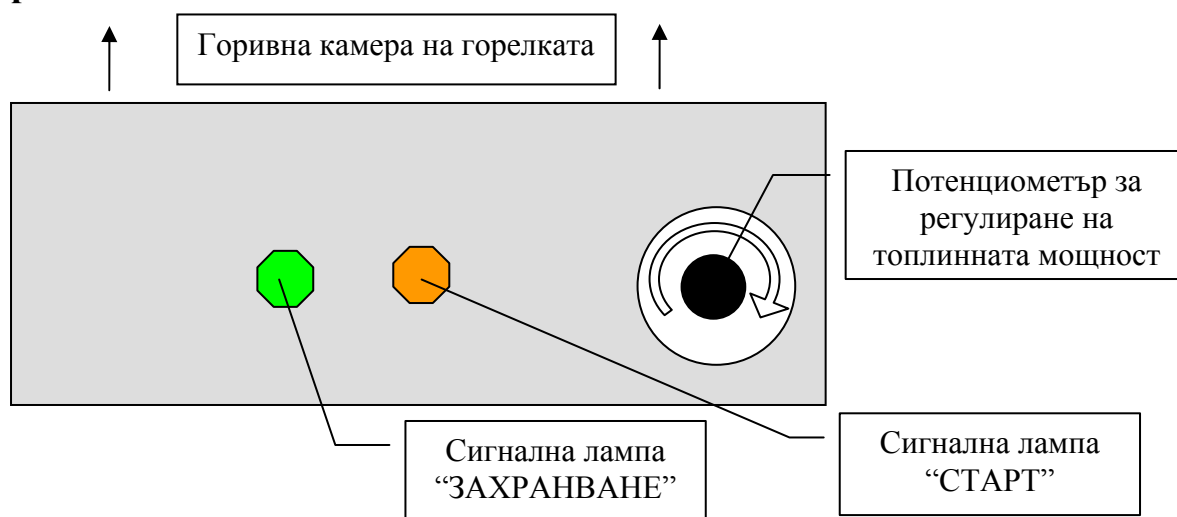
Фигура 5.1. Интерфейсно табло със сигнални лампи, контролни и управляващи уреди на автоматизирана горелка за пелети от серията “GP”.
