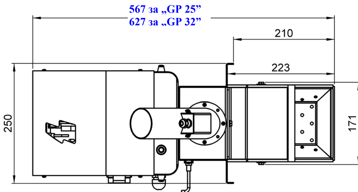
Фигура 4.3.3. Габаритни размери на основния модул на горелката от серията “GP” – поглед отгоре;
