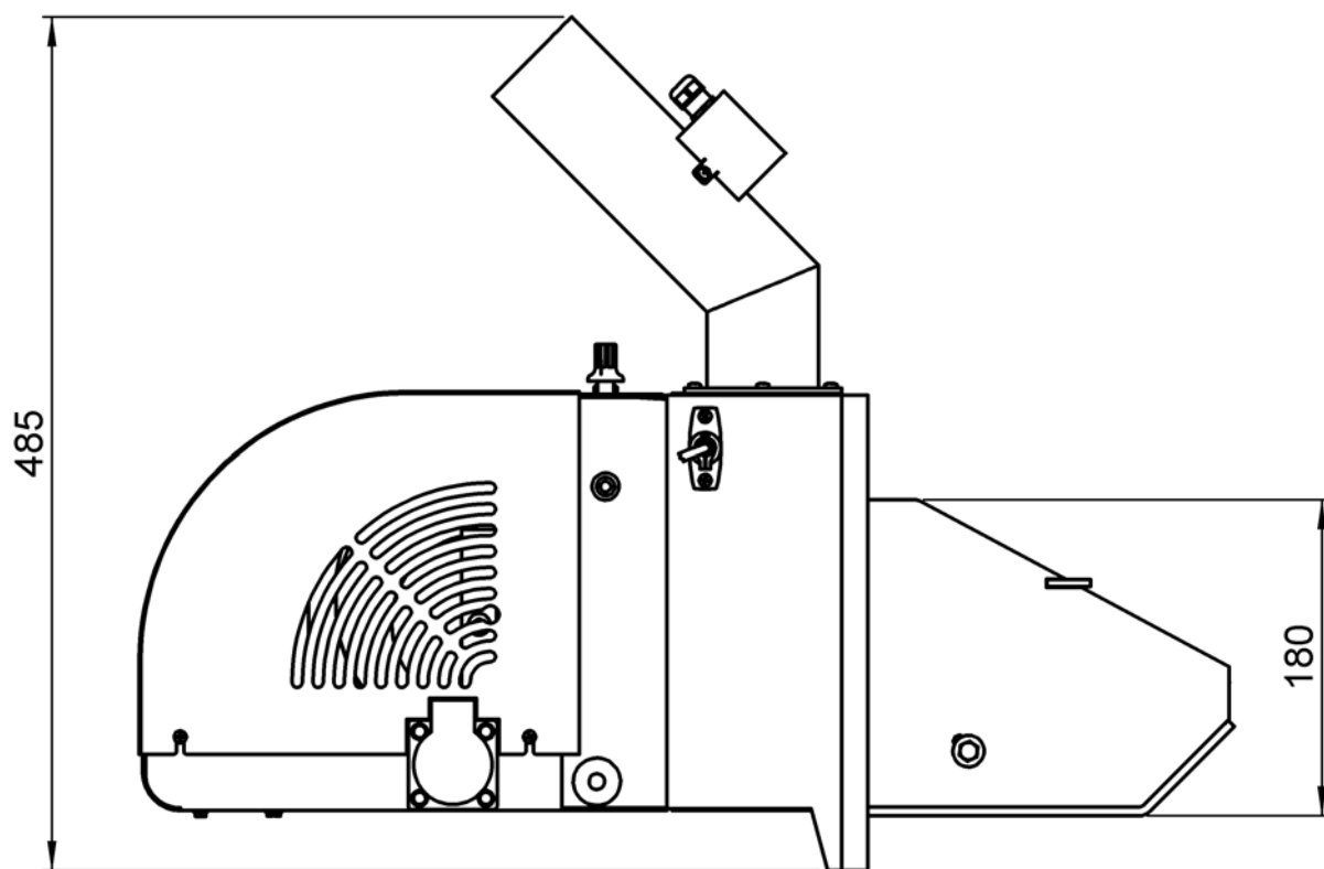
Фигура 4.3.2. Габаритни размери на основния модул на горелката от серията “GP” – поглед от страни;
