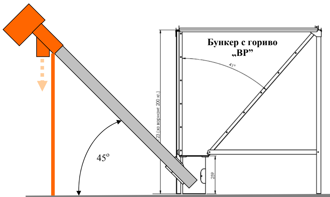
Фигура 4.3.5. Принципна схема за монтаж и разположение на гориво-подаващия транспортен шнек ( оста на шнека трябва да бъде под ъгъл 45^{\circ} спрямо хоризонталната равнина );
